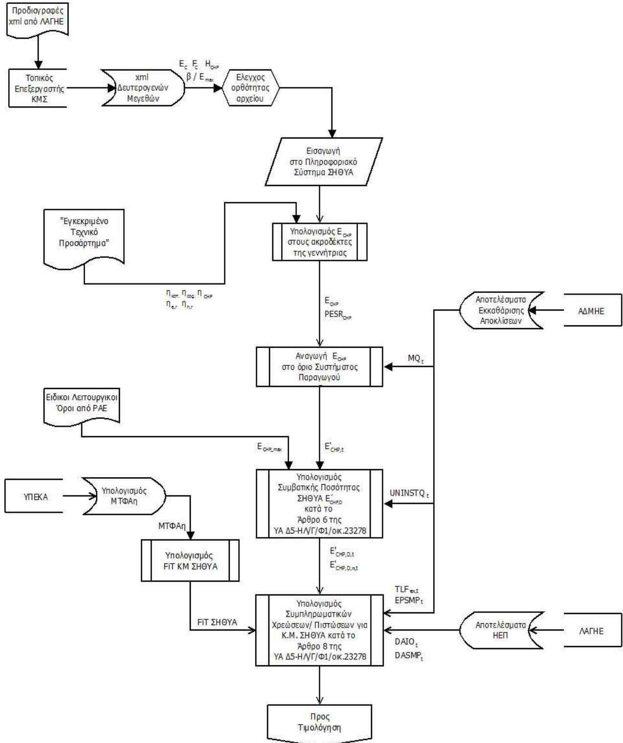
ΣΧΗΜΑ 34: Διαδικασία Συμπληρωματικής Εκκαθάρισης Μονάδων ΣΗΘΥΑ
