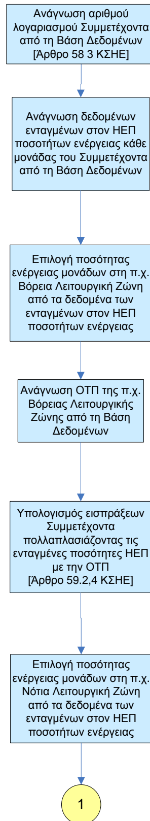
ΣΧΗΜΑ 11: ΗΕΠ51 – Υπολογισμοί Πληρωμών Εκκαθάρισης ΗΕΠ
