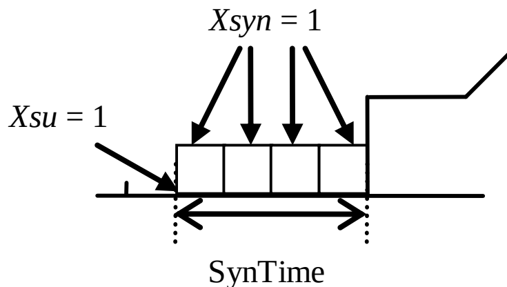
ΣΧΗΜΑ 27: Μοντελοποίηση Διαδικασίας Συγχρονισμού
