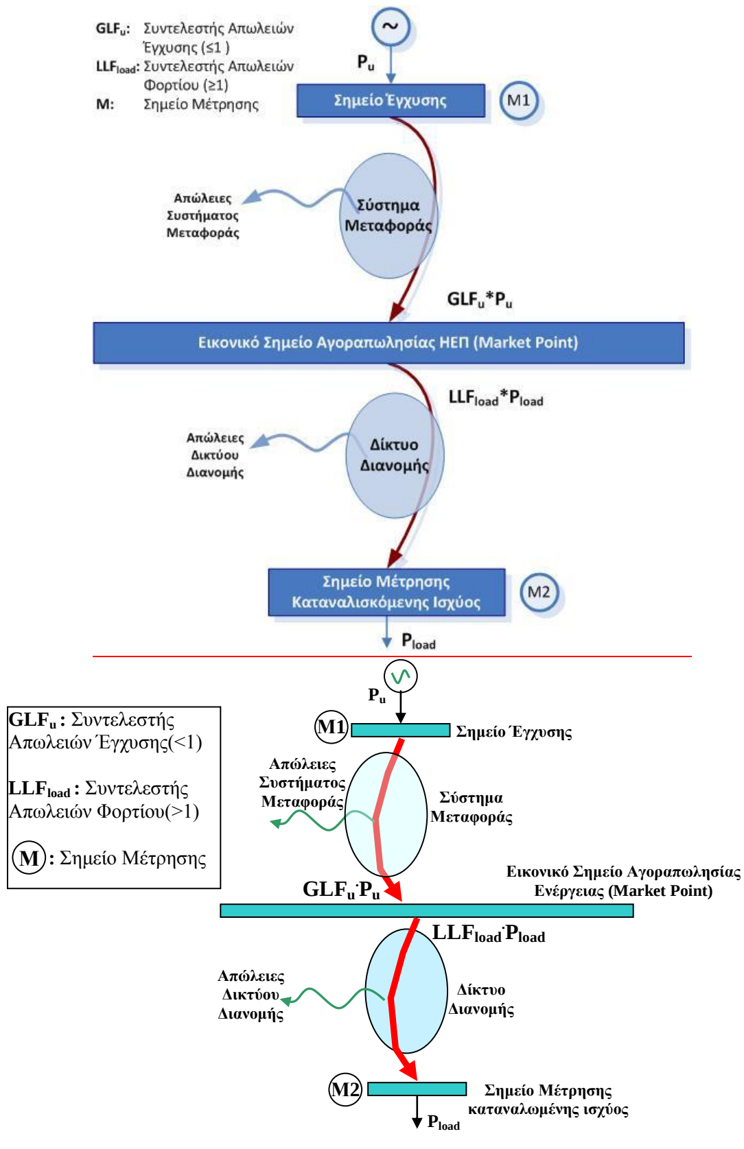
ΣΧΗΜΑ 2: Επίδραση των απωλειών μεταφοράς και διανομής
