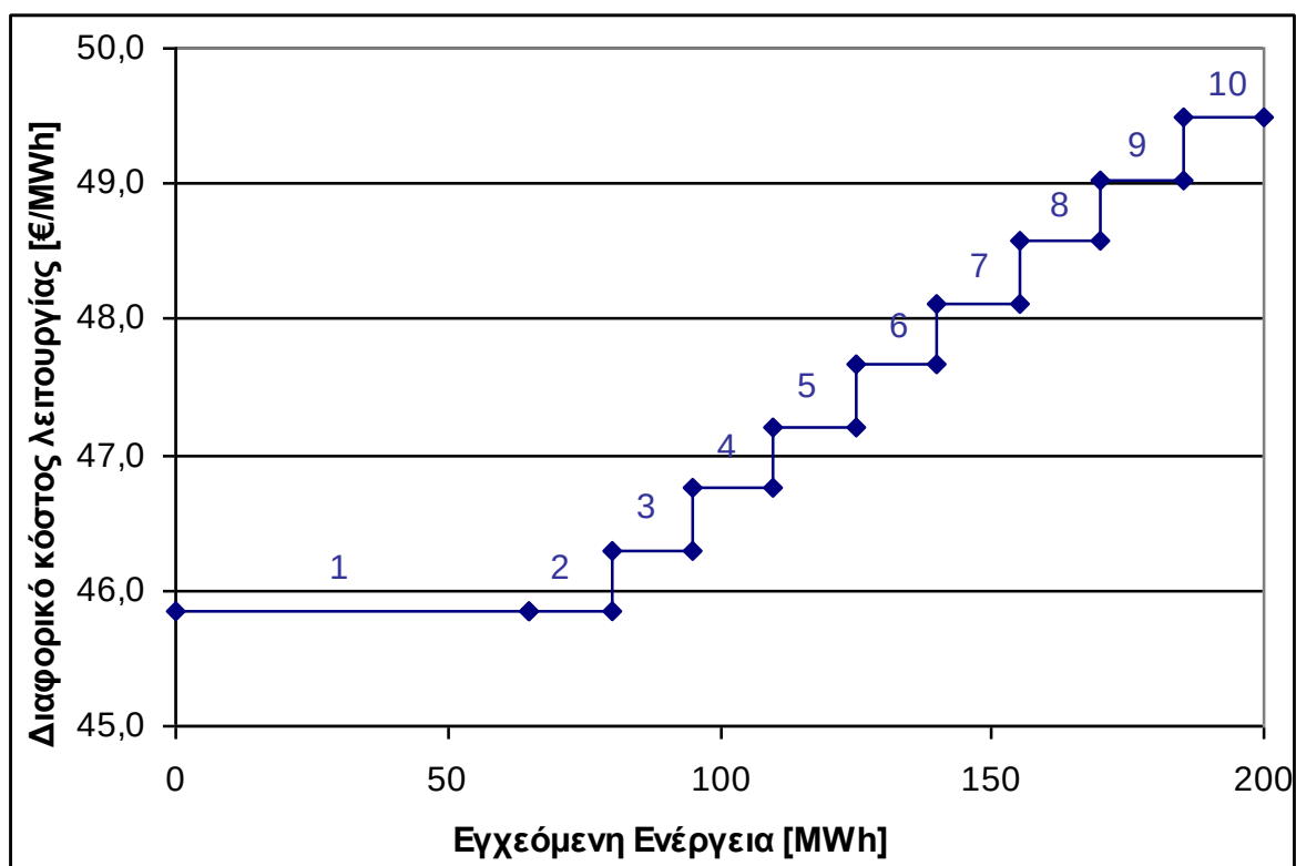
ΣΧΗΜΑ 21: Συνάρτηση Διαφορικού Κόστους της μ Mονάδας από 0 έως P_{max}
