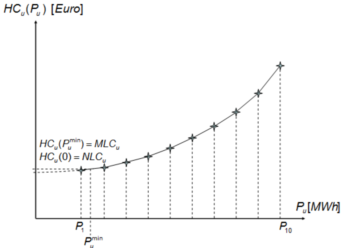
ΣΧΗΜΑ 18: Ωριαίο Κόστος Λειτουργίας θερμικής μ Μονάδας u
