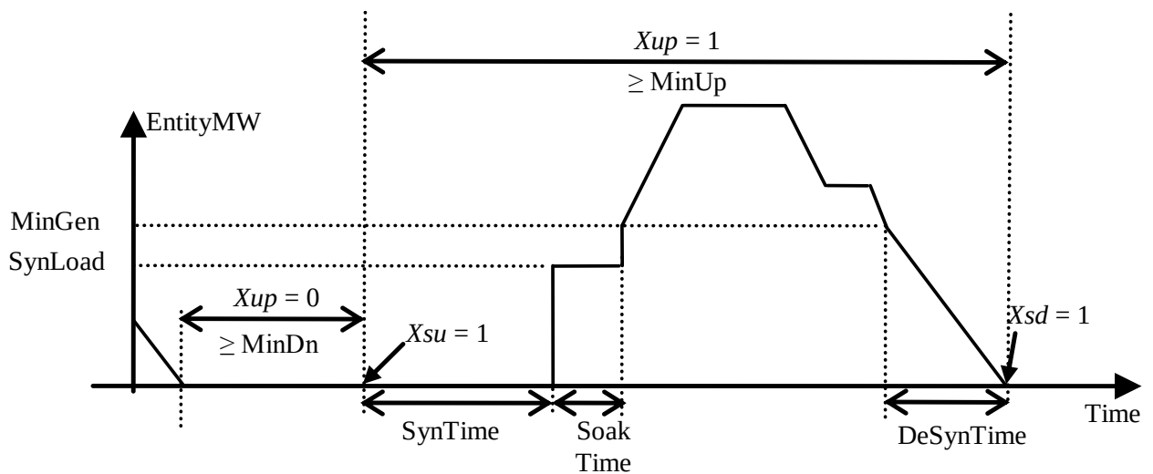
ΣΧΗΜΑ 26: Μοντελοποίηση Διαδικασίας Εκκίνησης - Σβέσης
