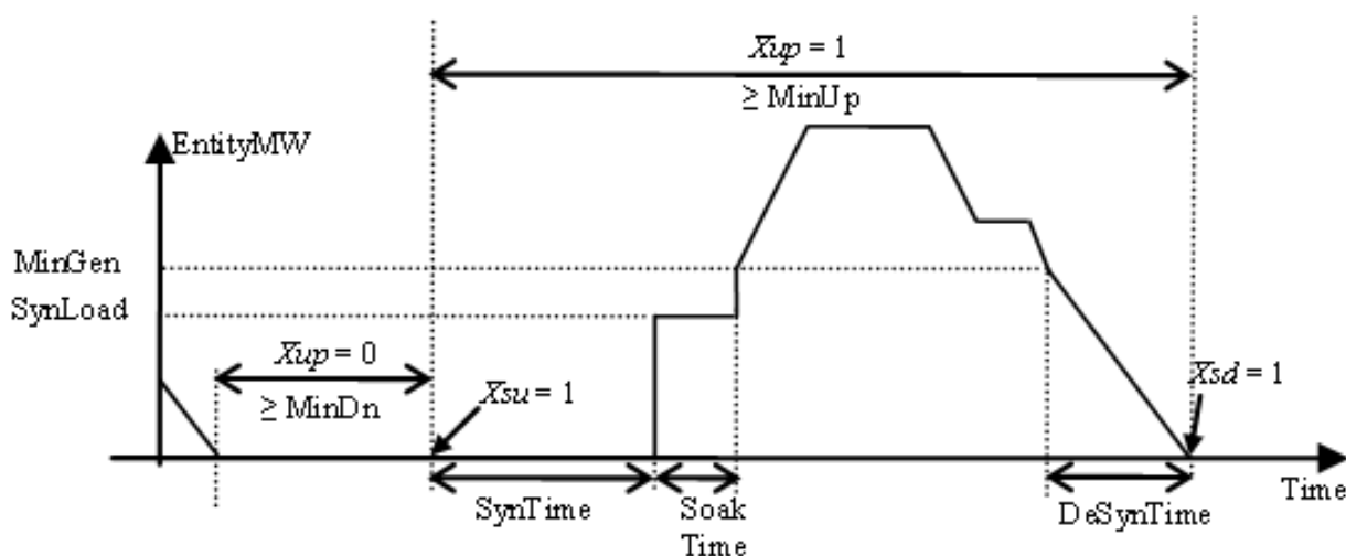
ΣΧΗΜΑ 25: Χρόνοι κύκλου λειτουργίας μΜονάδας
