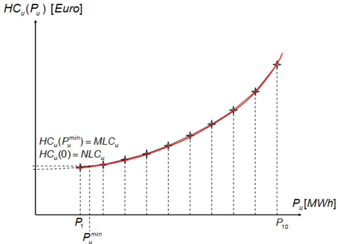
ΣΧΗΜΑ 19: Κλιμακωτή γραμμική προσέγγιση της καμπύλης Ωριαίου Κόστους Λειτουργίας
