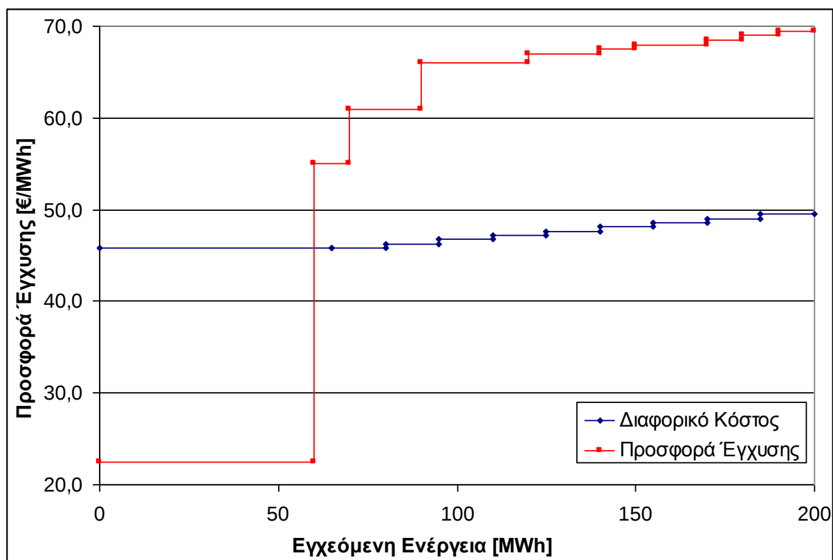
ΣΧΗΜΑ 25: Παράδειγμα Προσφοράς Έγχυσης Θερμικής Μονάδας
