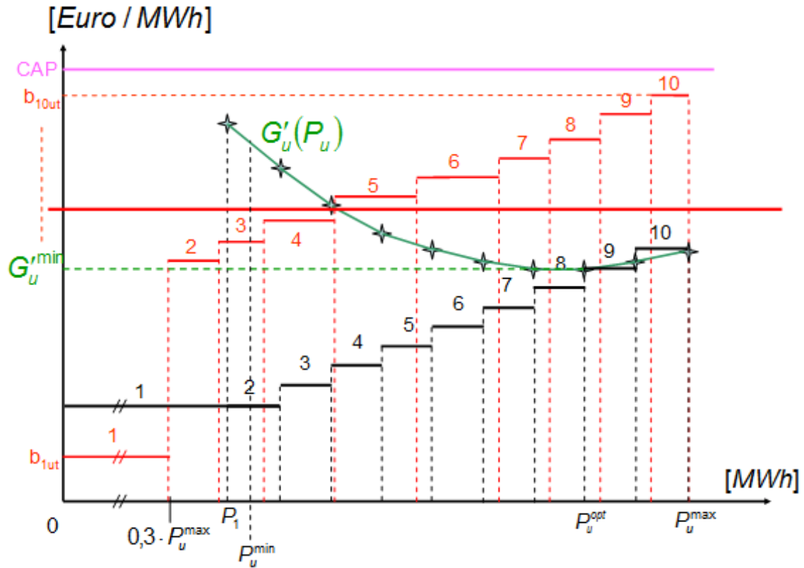
ΣΧΗΜΑ 22: Έλεγχος εγκυρότητας Προσφοράς Έγχυσης θερμικής Μονάδας
