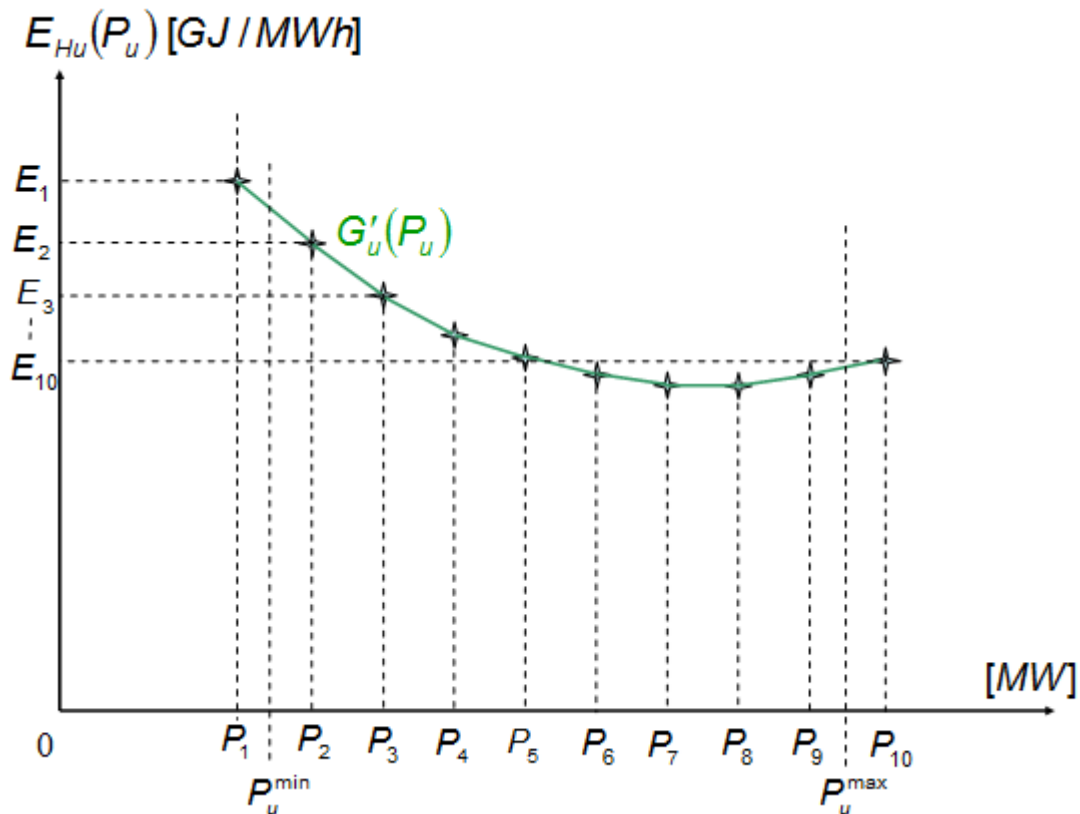
ΣΧΗΜΑ 16: Ειδική Κατανάλωση Θερμότητας Μονάδας u
