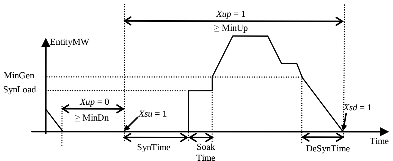
ΣΧΗΜΑ 27: Μοντελοποίηση Διαδικασίας Εκκίνησης - Σβέσης
