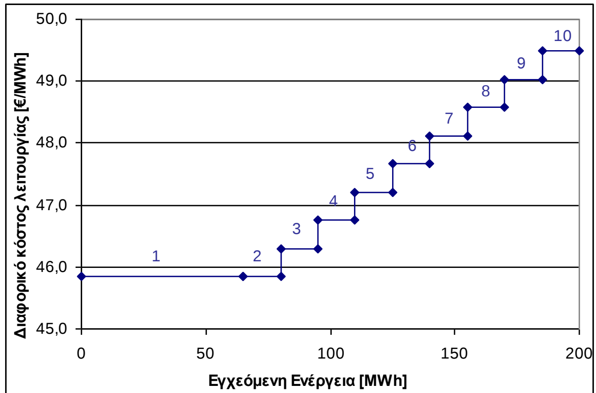
ΣΧΗΜΑ 21: Συνάρτηση Διαφορικού Κόστους της Μονάδας από 0 έως P_{max}
