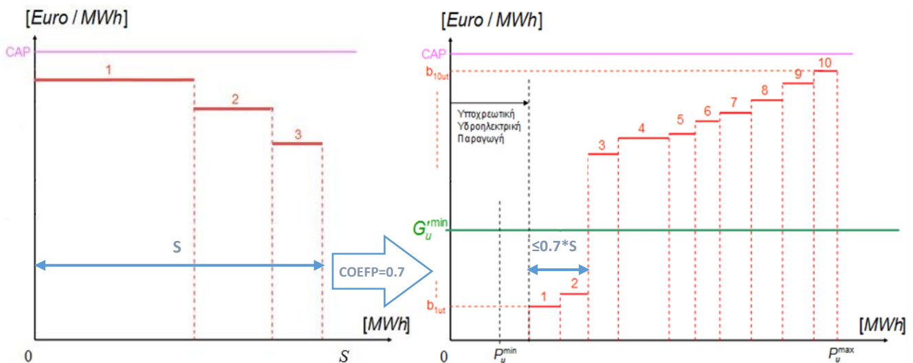
ΣΧΗΜΑ 24: Έλεγχος εγκυρότητας Προσφοράς Έγχυσης υδροηλεκτρικής Μονάδας η οποία έχει υποβάλλει Τιμολογούμενη Δήλωση Φορτίου για άντληση
