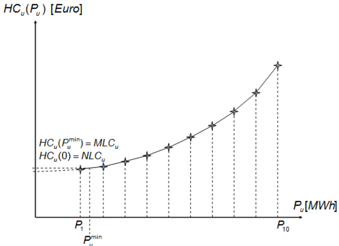
ΣΧΗΜΑ 18: Ωριαίο Κόστος Λειτουργίας θερμικής Μονάδας u
