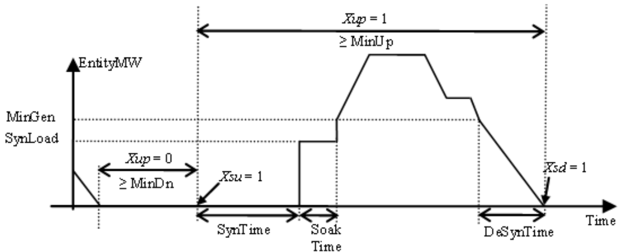
ΣΧΗΜΑ 26: Χρόνοι κύκλου λειτουργίας Μονάδας
