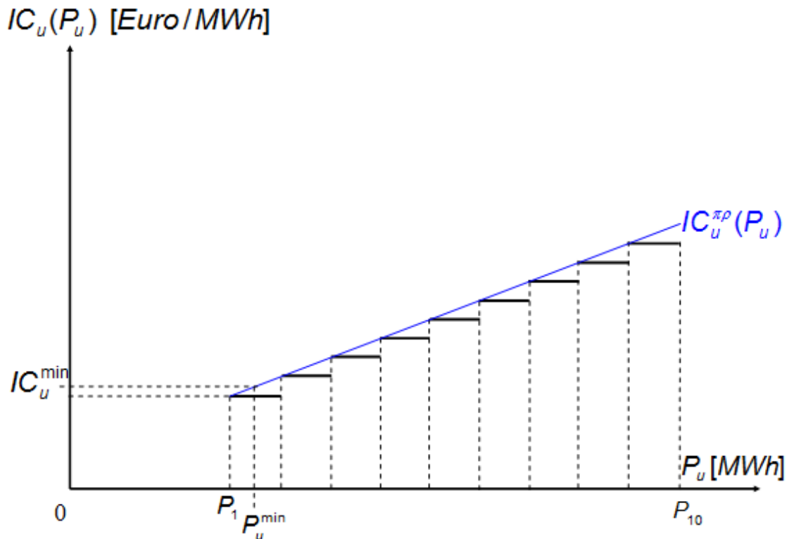
ΣΧΗΜΑ 20: Χαρακτηριστική καμπύλη Διαφορικού Κόστους θερμικής Μονάδας u
