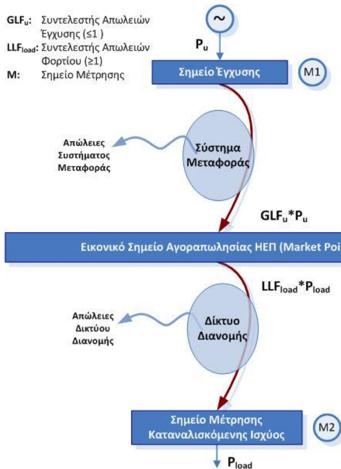
ΣΧΗΜΑ 2: Επίδραση των απωλειών μεταφοράς και διανομής
