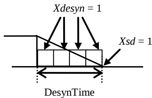
ΣΧΗΜΑ 30: Μοντελοποίηση Διαδικασίας Αποσυγχρονισμού
